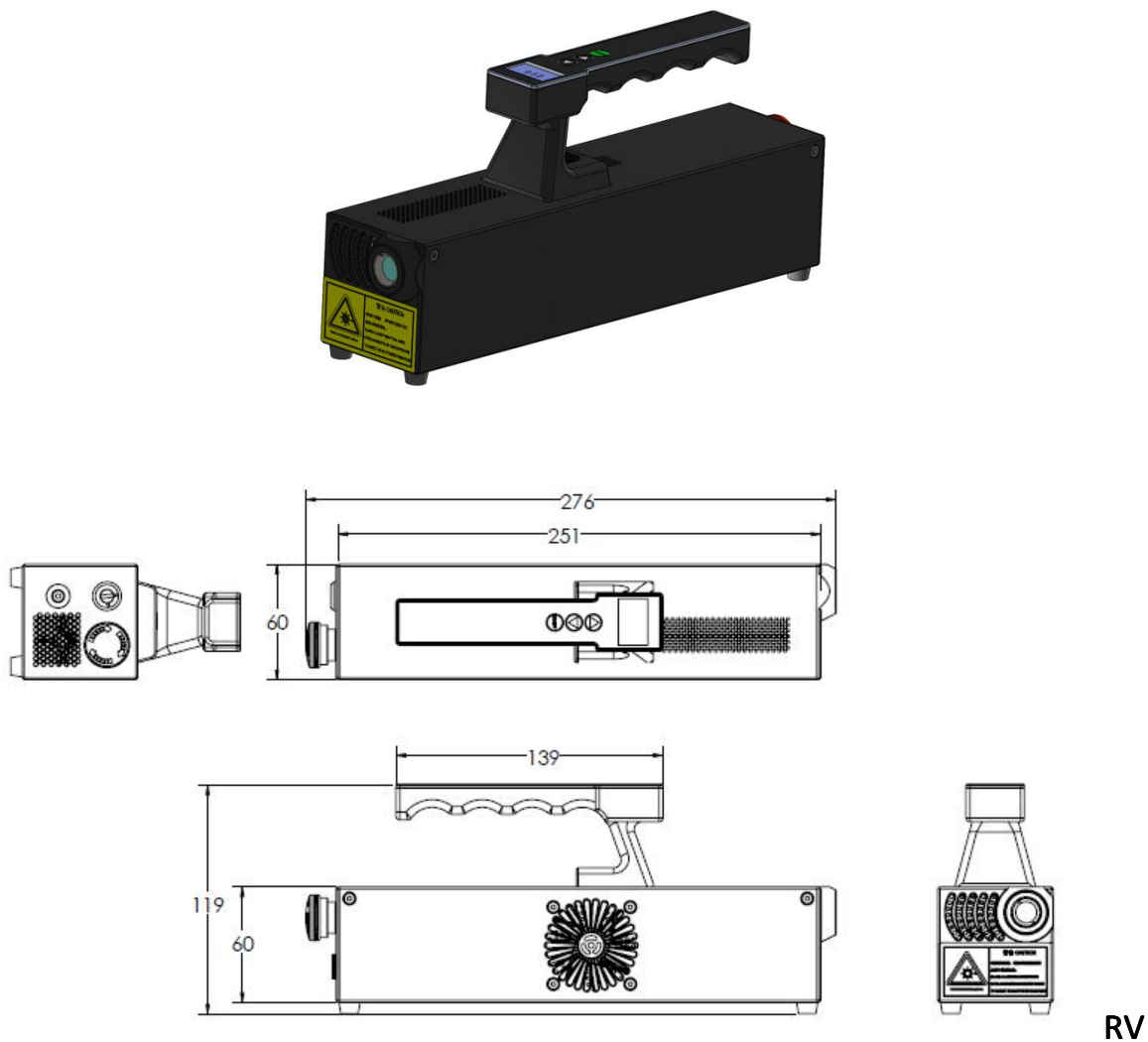
ZBD-BG-9030H/ZBD-B-12H/ZBD-G-40H结构尺寸图
